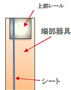
断面取付図
