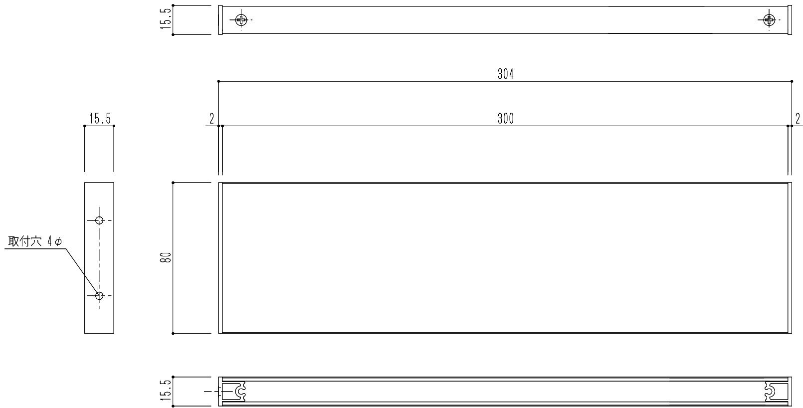
断面図
