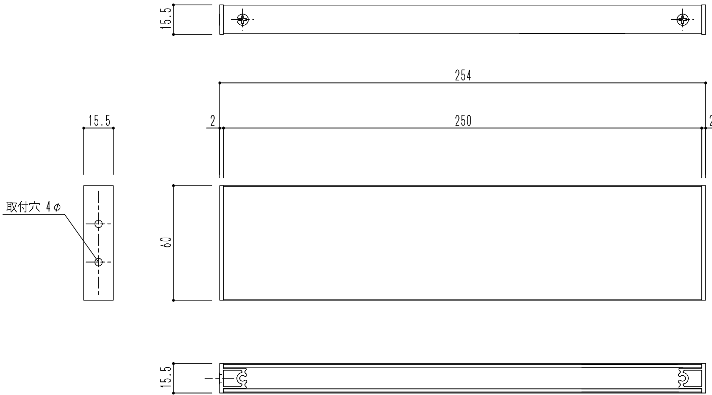
断面図
