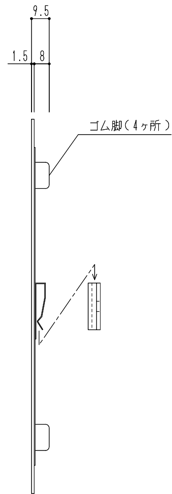
取付金具
