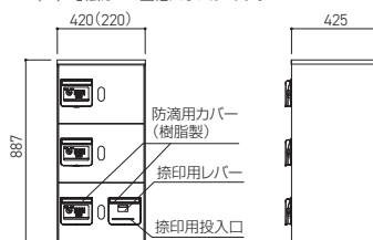
図例 SK-CBX-402型 ※ ( ) 寸法は702型他スリムタイプ。
