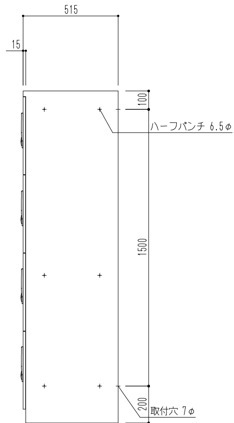
側面図
