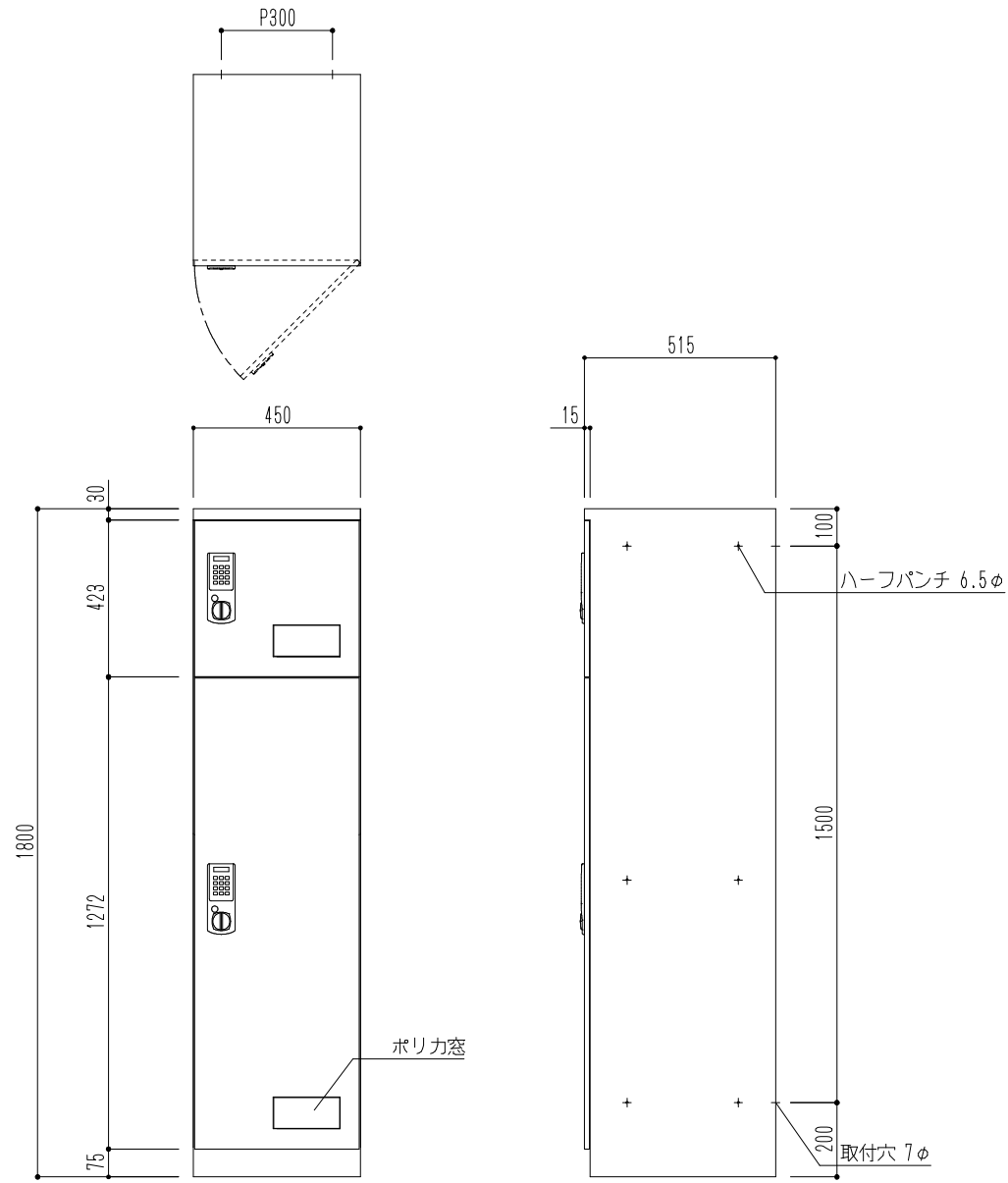
側面図
