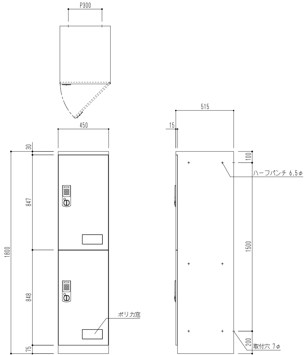
側面図
