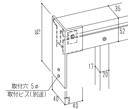
取付金具
