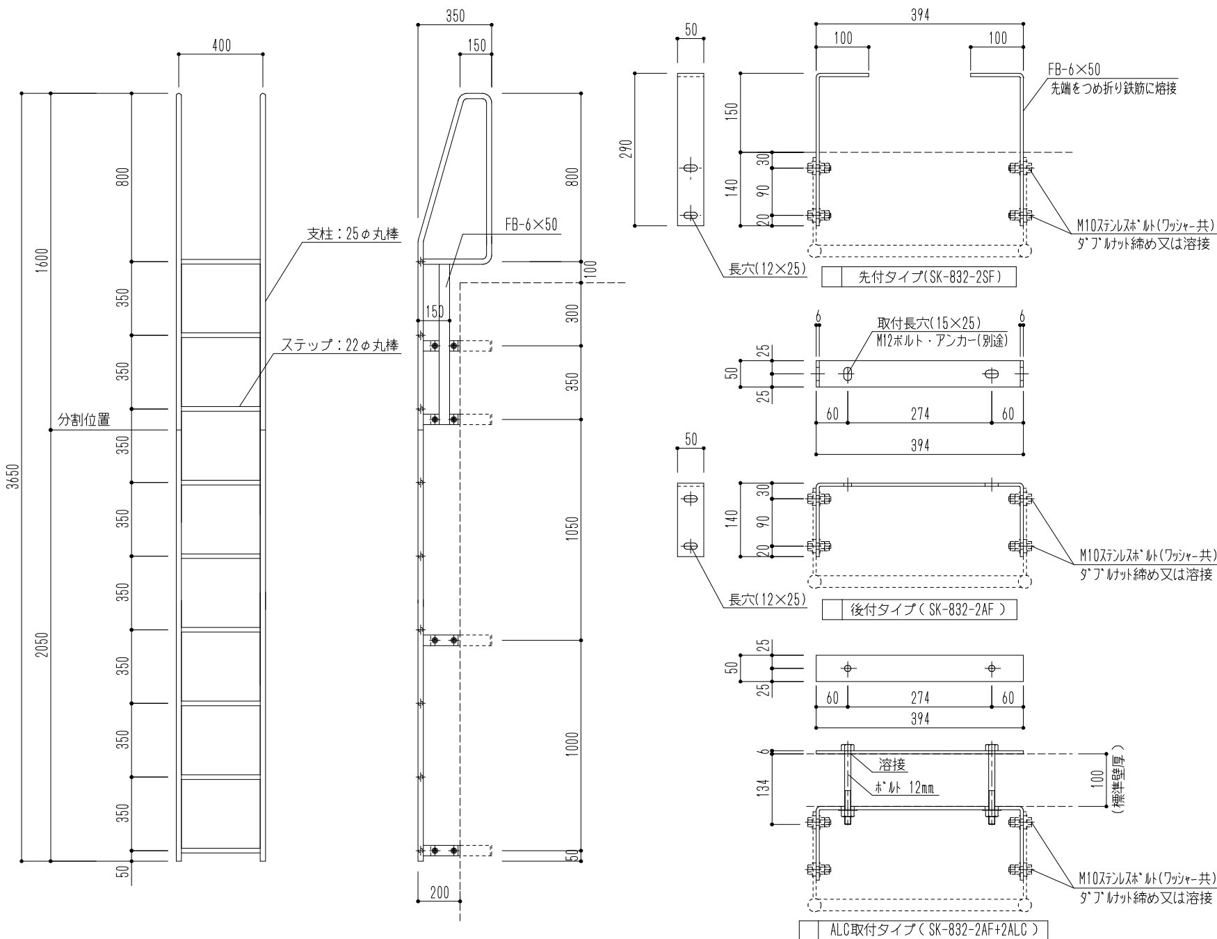
図面名 SK-832N-2 塔屋タラップ
