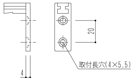
座金詳細
