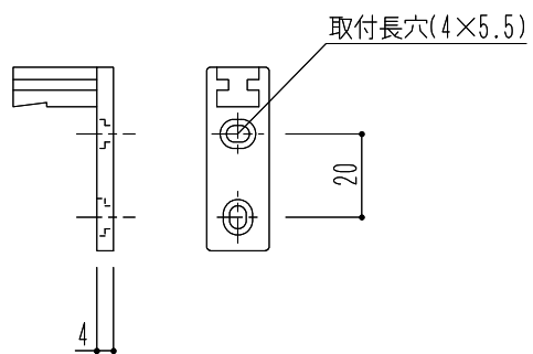
座金詳細
