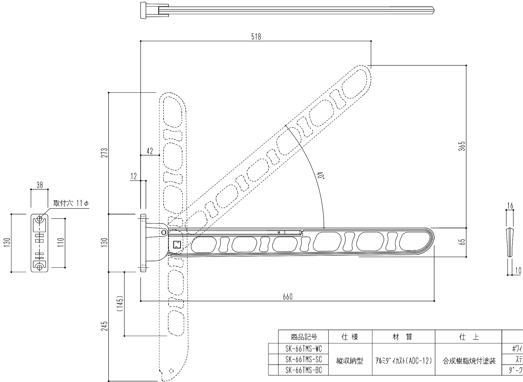
図面名 SK-66TMS-WC/-SC/-BC アルミダイカスト物干金物(縦収納型)
