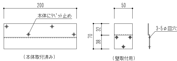
取付ブラケット詳細図
