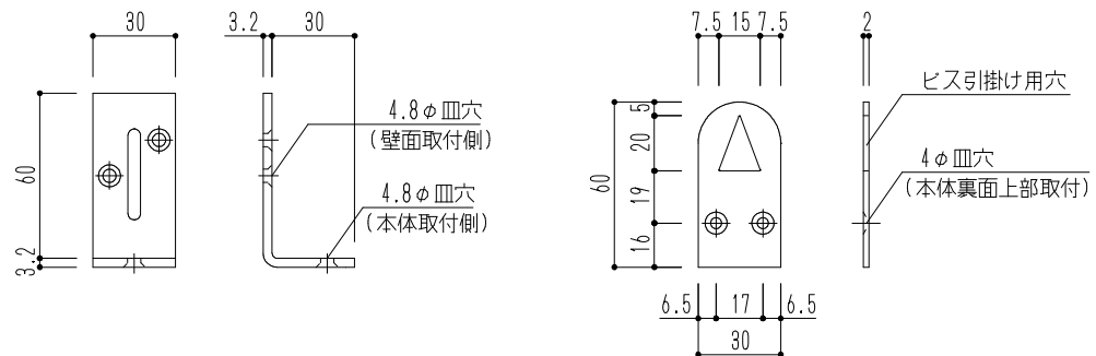
取付金具
