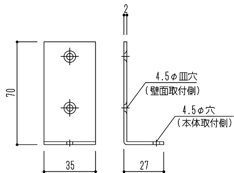
取付金具
