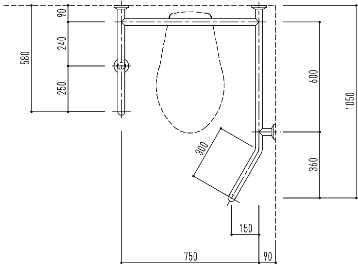
右勝手(R)
